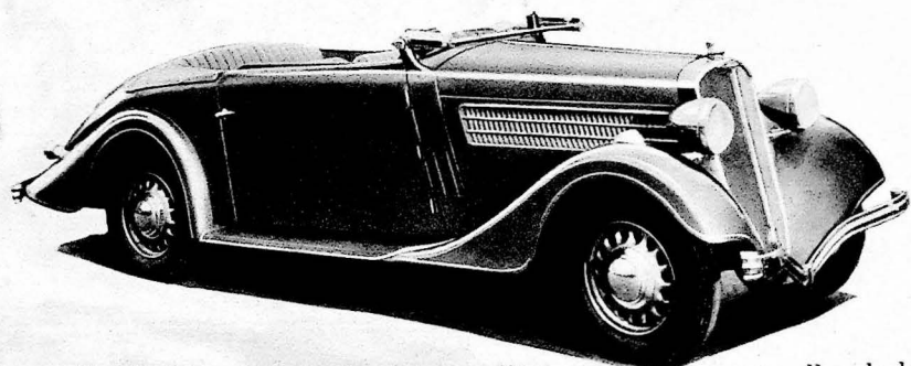
Une conduite intérieure SALMON et un élégant roadster luxe de ligne très sportive sur le châssis 10 CV. S. 4 D. A. dont on connaît le fameux moteur double arbre à cames en tête, au rendement exceptionnel et d'une économie proverbiale. Salomon sort pour le Salon une nouvelle 13 CV. à boîte COTAL, voiture grande routière qui aura vite son public.
